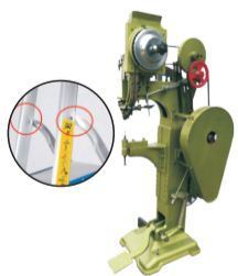
铆钉机 RIVET MACHINE
