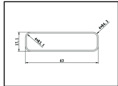
DY-Balance Bar SQB020
