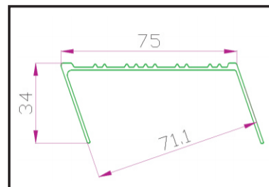
踏板 Step Profile
